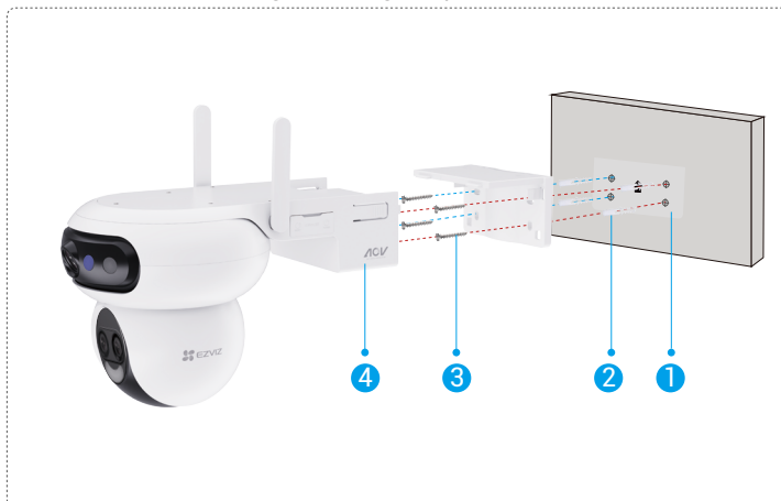
Fig. 2 Montage mural
